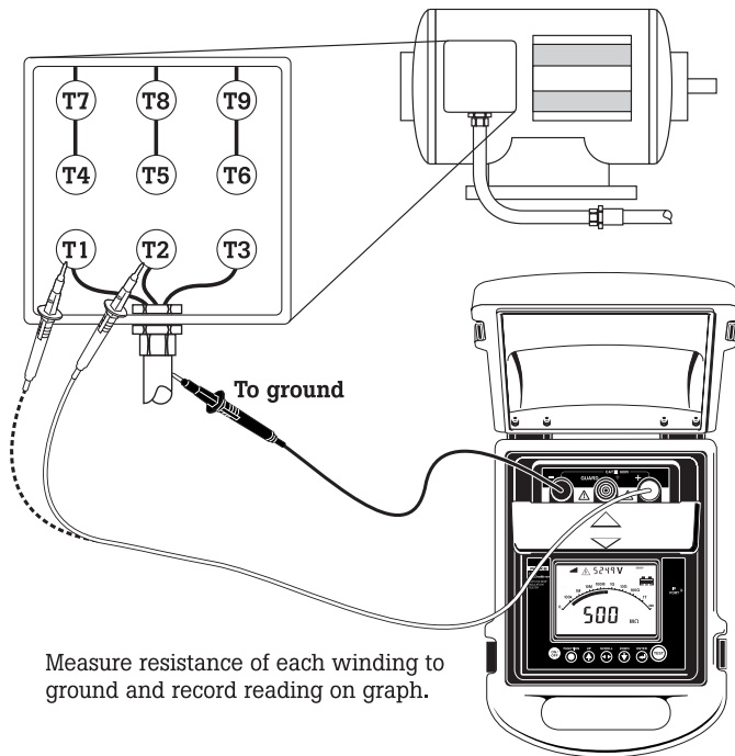
Megohmmeter
